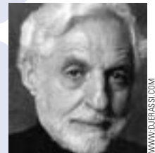
Carl Djerassi
